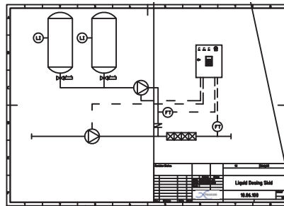
Voorbeeld P&ID van een doseersysteem
