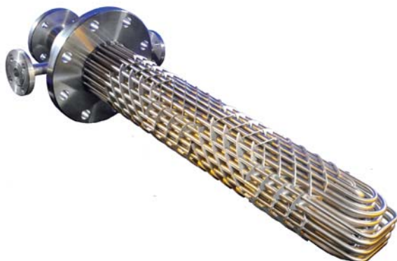
CSE-XR mixer warmtewisselaar
