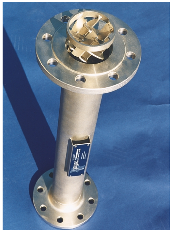
Fig. 5: Fluitec mixer CSE-X
